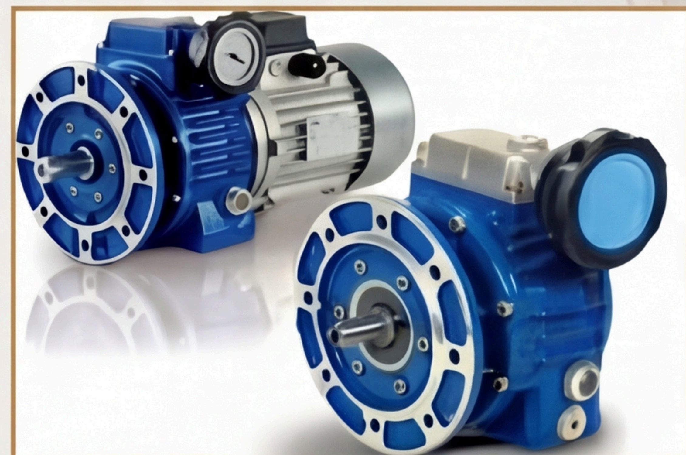
VARIATEUR MÉCANIQUE
